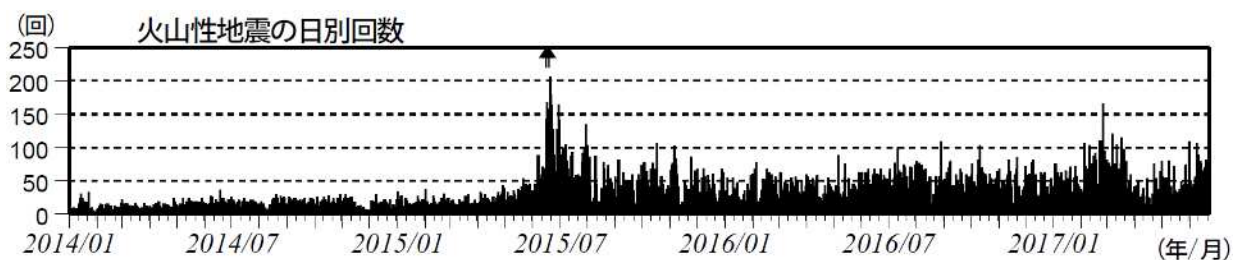
図2 浅間山 火山性地震の日別回数（2014年1月1日～2017年6月22日） （矢印はごく小規模な噴火を示す）
