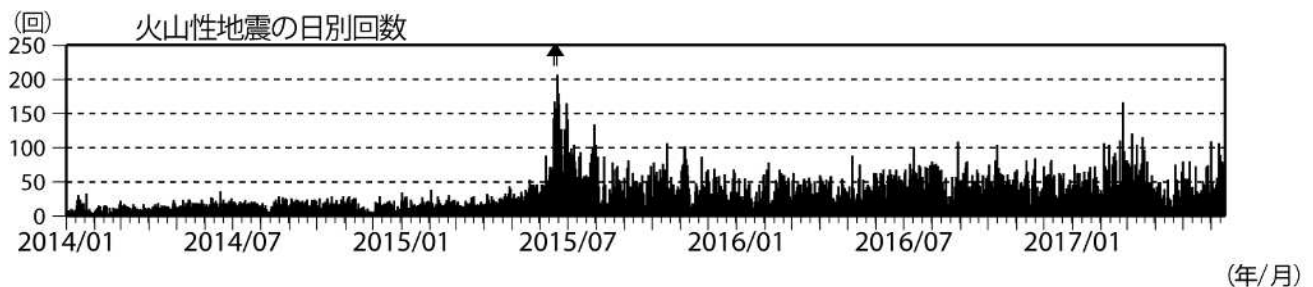
図2 浅間山 火山性地震の日別回数（2014年1月1日～2017年6月15日） （矢印はごく小規模な噴火を示す）
