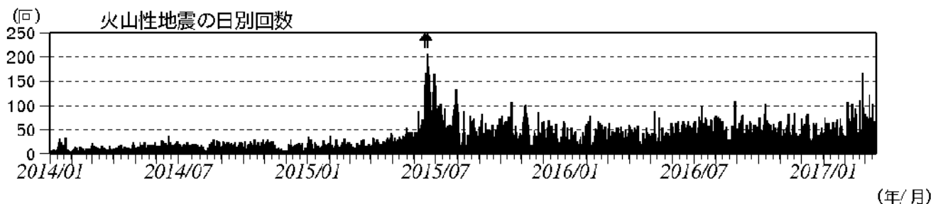
図2 浅間山 火山性地震の日別回数（2014年1月1日～2017年3月16日） （矢印はごく小規模な噴火を示す）
