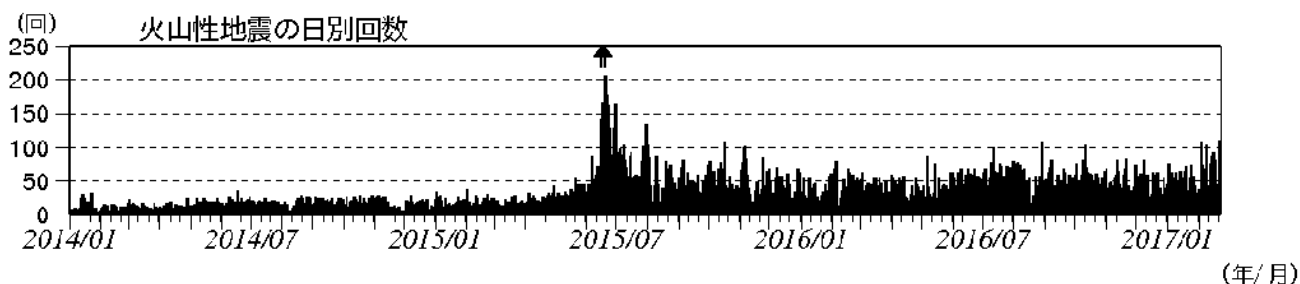
図2 浅間山 火山性地震の日別回数（2014年1月1日～2017年2月23日） （矢印はごく小規模な噴火を示す）
