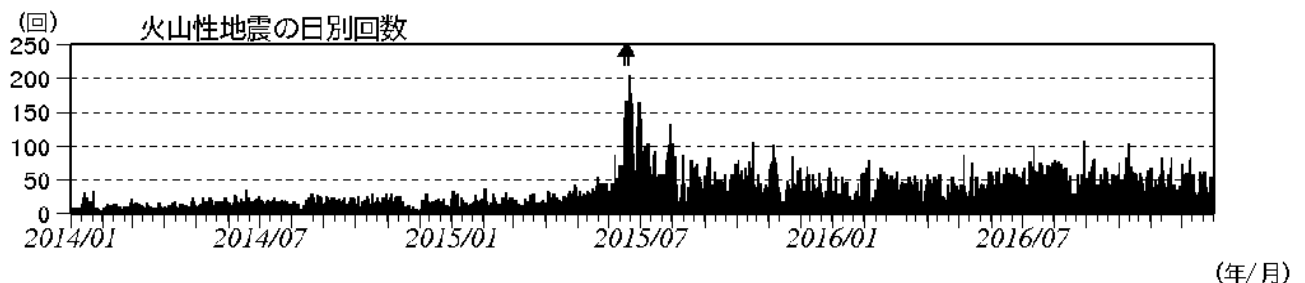
図2 浅間山 火山性地震の日別回数（2014年1月1日～2016年12月29日） （矢印はごく小規模な噴火を示す）
