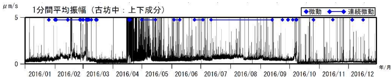
図3 阿蘇山 古坊中観測点上下成分の1分間平均振幅(2016年1月1日~2016年12月29日)
