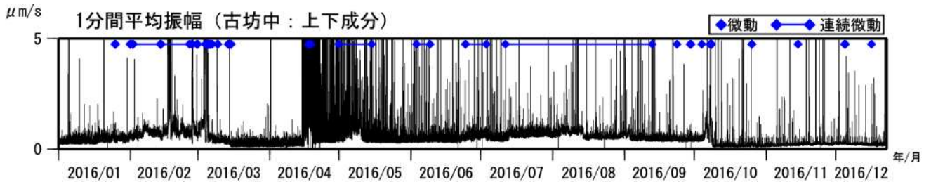
図3 阿蘇山 古坊中観測点上下成分の1分間平均振幅(2016年1月1日~2016年12月22日)
