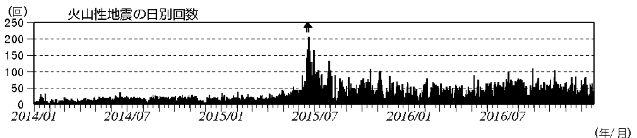
図2 浅間山 火山性地震の日別回数（2014年1月1日～2016年12月22日） （矢印はごく小規模な噴火を示す）
