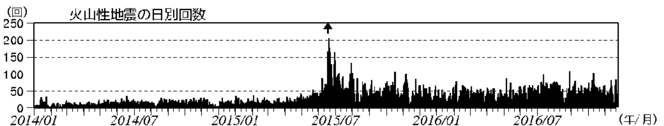
図2 浅間山 火山性地震の日別回数（2014年1月1日～2016年11月24日） （矢印はごく小規模な噴火を示す）
