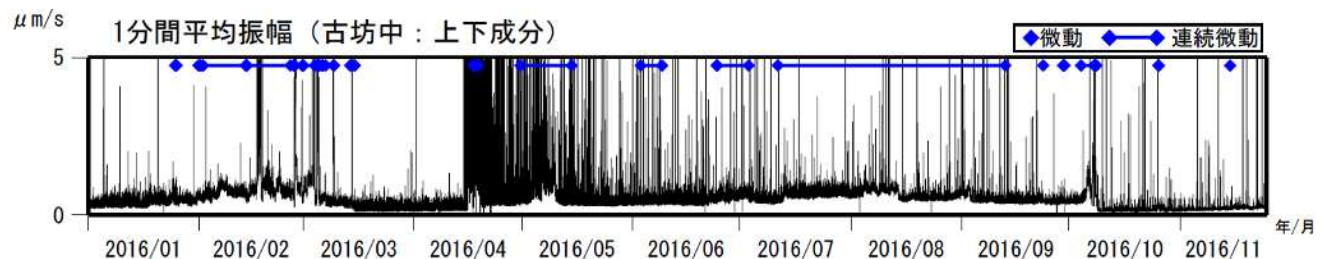
図3 阿蘇山 古坊中観測点上下成分の1分間平均振幅 (2016年1月1日~2016年11月24日)
