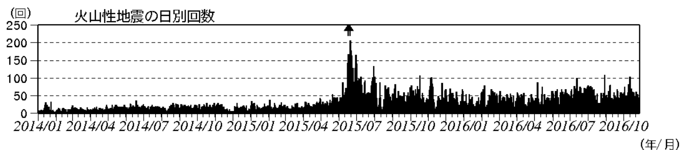
図 2 浅間山 火山性地震の日別回数（2014 年 1 月 1 日～2016 年 10 月 27 日） （矢印はごく小規模な噴火を示す）
