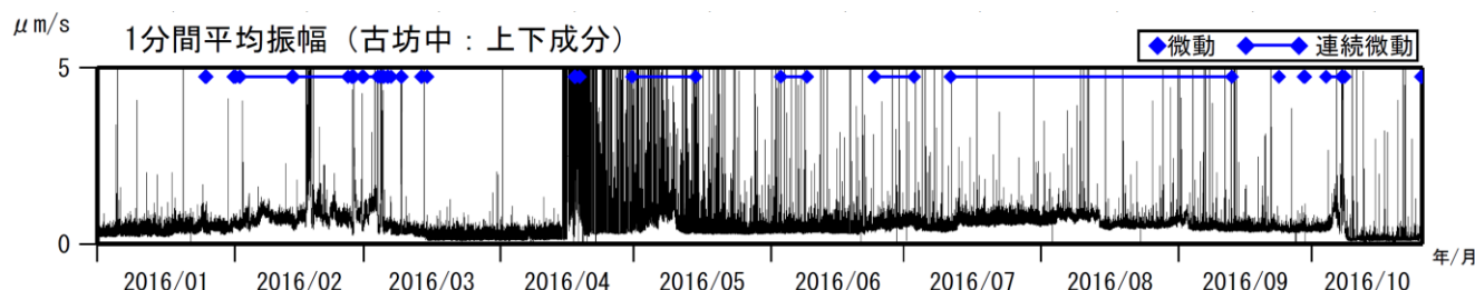
図3 阿蘇山 古坊中観測点上下成分の1分間平均振幅（2016年1月1日～2016年10月27日）
