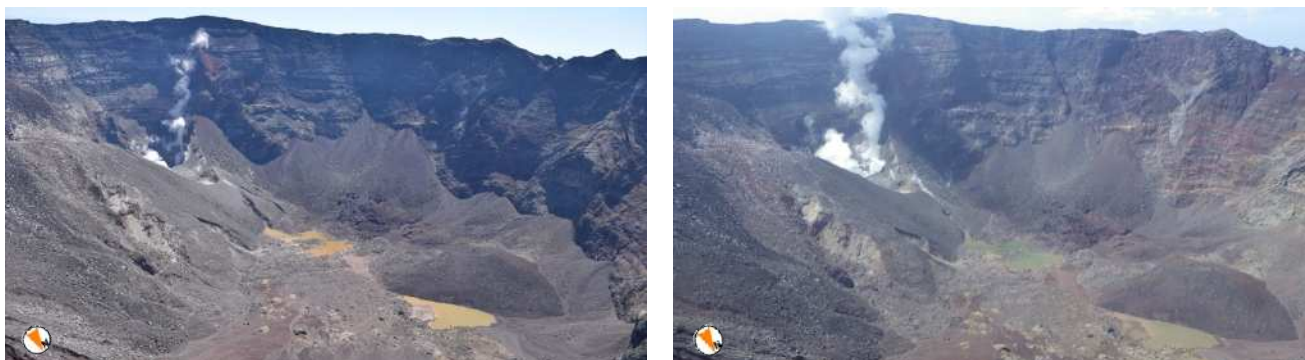
図 5 三宅島 山頂火口内の状況（左：2016 年 5 月 12 日、右：2016 年 4 月 6 日）
