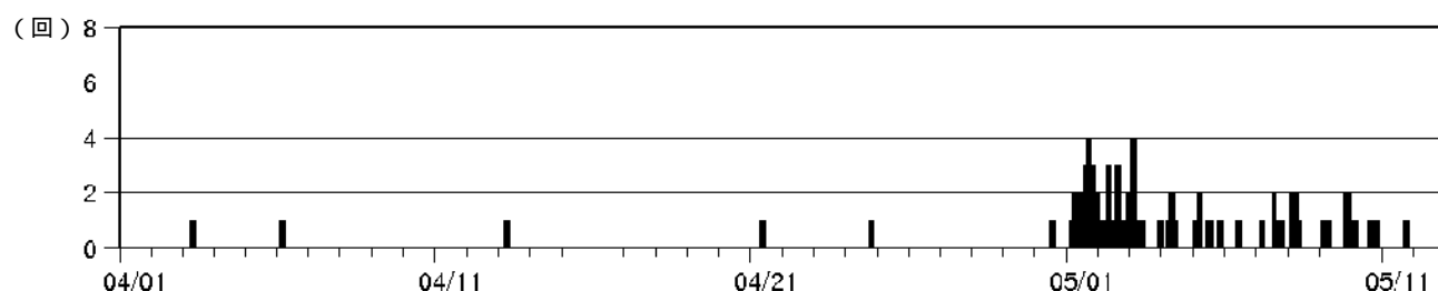
時間別 低周波地震 11) 回数
