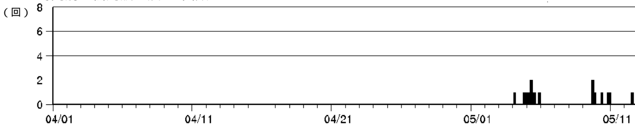
図4 新潟焼山 火山性地震の時間別回数(2016年4月1日~2016年5月12日)
