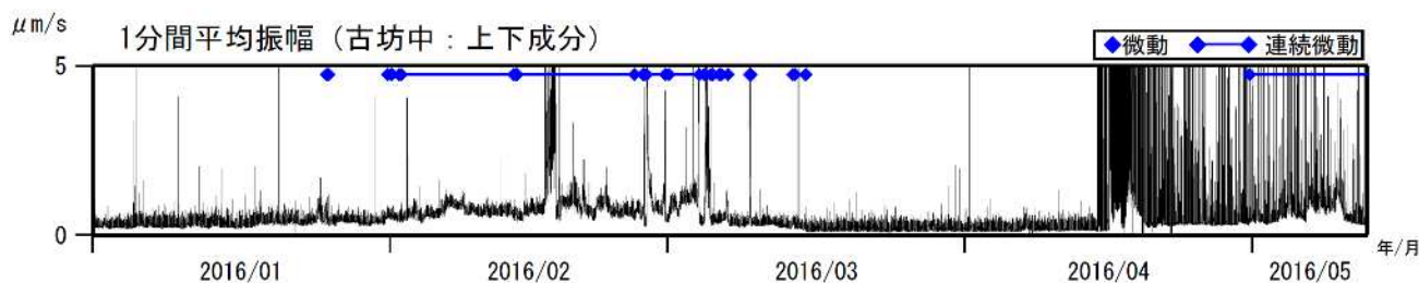
図3 阿蘇山 古坊中観測点上下成分の1分間平均振幅(2016年1月1日～2016年5月12日)
