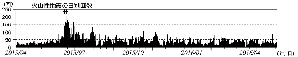
図2 浅間山 火山性地震の日別回数（2015年4月1日～2016年5月12日）（矢印はごく小規模な噴火を示す）
