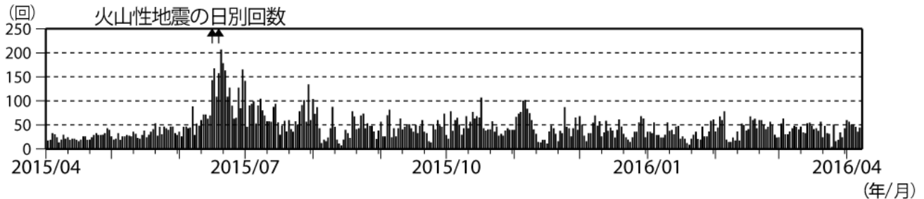
図 3 浅間山 火山性地震の日別回数（2015 年 4 月 1 日～2016 年 4 月 7 日）（矢印はごく小規模な噴火を示す）
