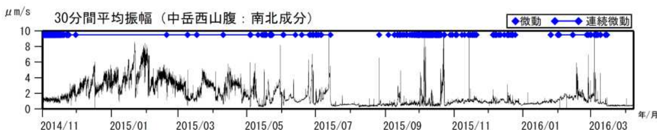
図4 阿蘇山 火山性微動の30分間平均振幅（2014年11月1日～2016年4月7日）
