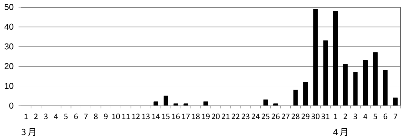
図2 吾妻山 火山性地震の日別回数（2016年3月1日～4月7日）
