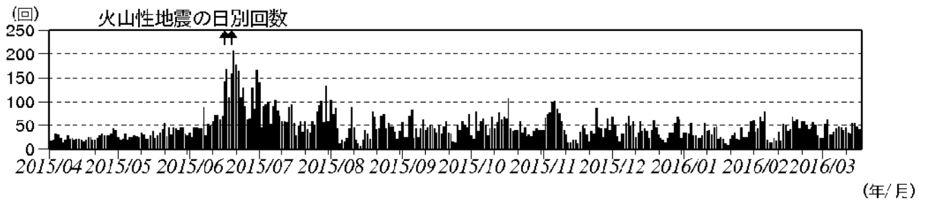
図2 浅間山 火山性地震の日別回数(2015年4月1日~2016年3月17日)(矢印はごく小規模な噴火を示す)
