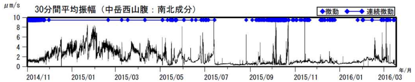
図3 阿蘇山 火山性微動の30分間平均振幅(2014年11月1日~2016年3月17日)
