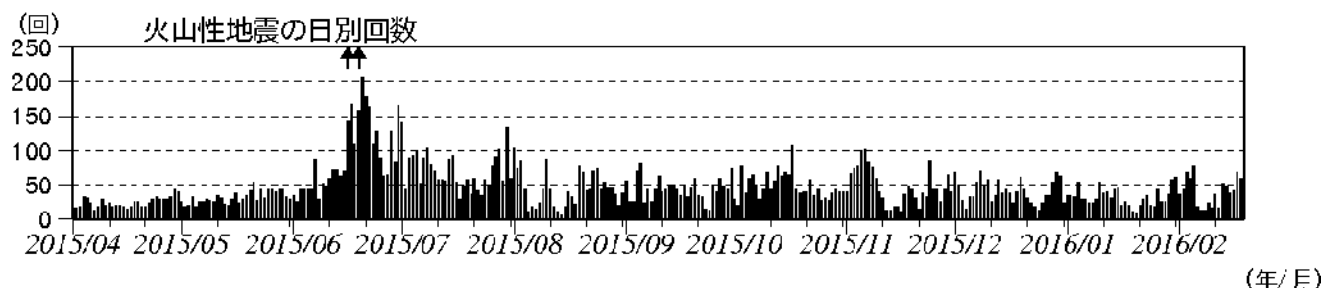
図2 浅間山 火山性地震の日別回数 (2015年4月1日～2016年2月18日) (矢印はごく小規模な噴火を示す)
