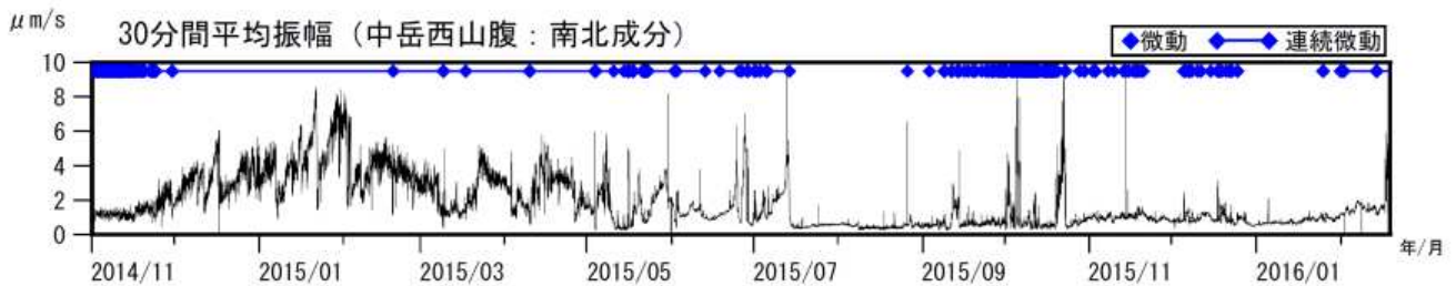
図3 阿蘇山 火山性微動の30分間平均振幅（2014年11月1日～2016年2月18日）
