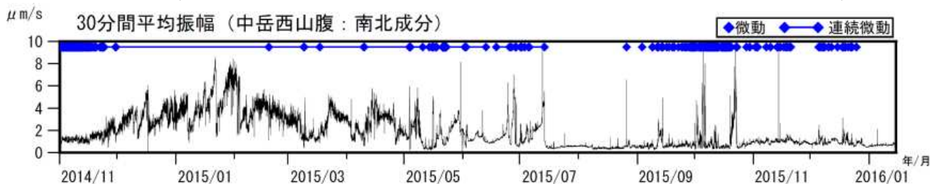
図3 阿蘇山 火山性微動の30分間平均振幅（2014年11月1日～2016年1月14日）
