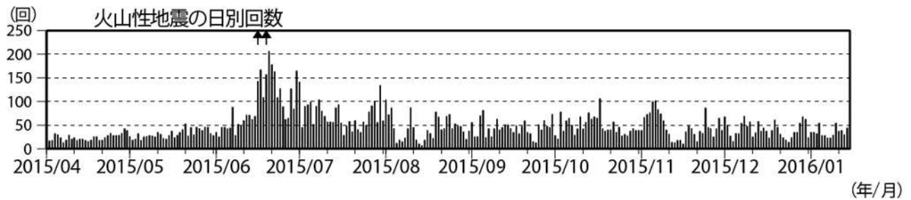
図2 浅間山 火山性地震の日別回数（2015年4月1日～2016年1月14日）（矢印はごく小規模な噴火を示す）
