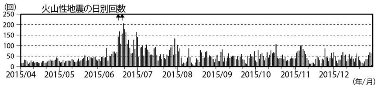
図2 浅間山 火山性地震の日別回数（2015年4月1日～12月31日）（矢印はごく小規模な噴火を示す）
