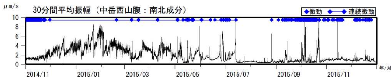
図3 阿蘇山 火山性微動の30分間平均振幅（2014年11月1日～2015年12月31日）
