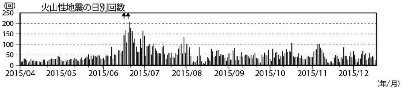
図2 浅間山 火山性地震の日別回数(2015年4月1日～12月17日)(矢印はごく小規模な噴火を示す)
