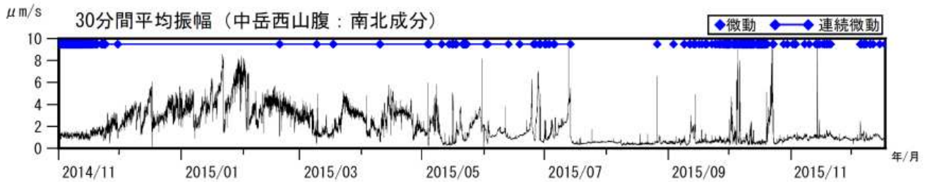
図3 阿蘇山 火山性微動の30分間平均振幅（2014年11月1日～2015年12月17日）
