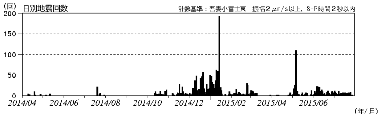
図 3 吾妻山 火山性地震の発生状況（2014 年 4 月 1 日～2015 年 7 月 30 日）
