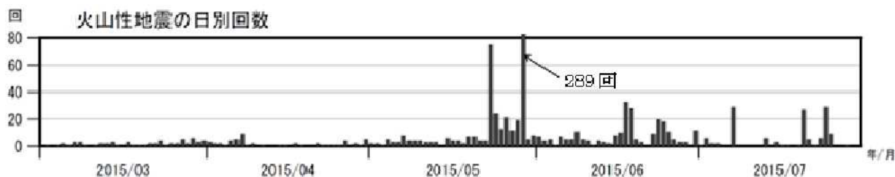
図7 口永良部島 火山性地震の日別回数（2015年3月1日～7月30日）
