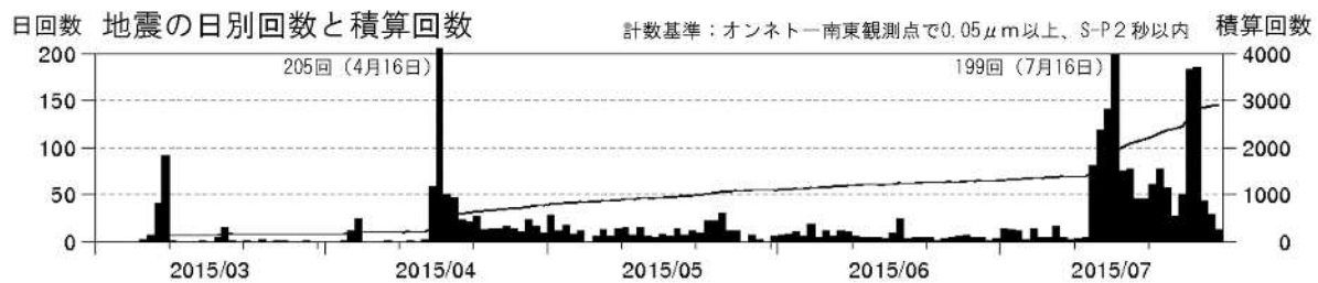
図 2 雌阿寒岳 火山性地震の発生状況（日回数及び積算回数 2015 年 3 月 1 日～7 月 30 日）
