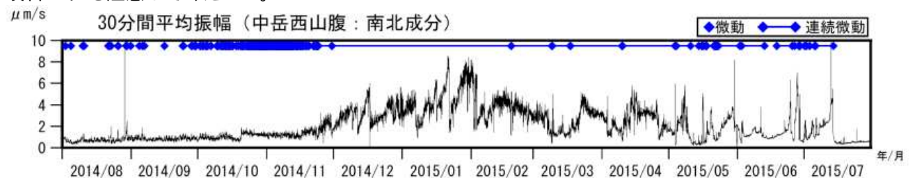
図6 阿蘇山 火山性微動の30分間平均振幅（2014年8月1日～2015年7月30日）
