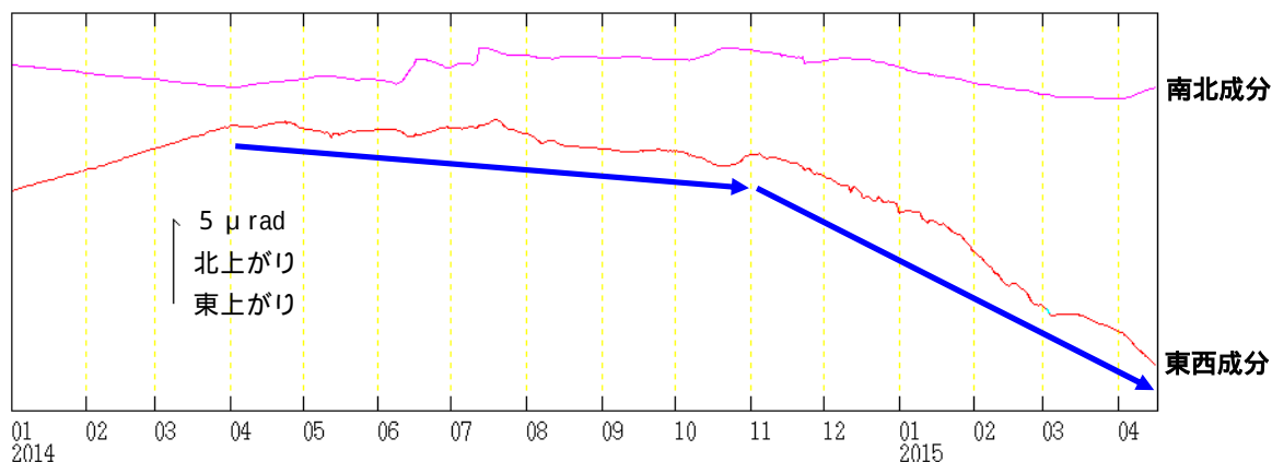
図4 吾妻山 浄土平観測点での傾斜変動（2014年1月1日～2015年4月16日） →は、傾斜変動傾向（東西成分）を示します。
