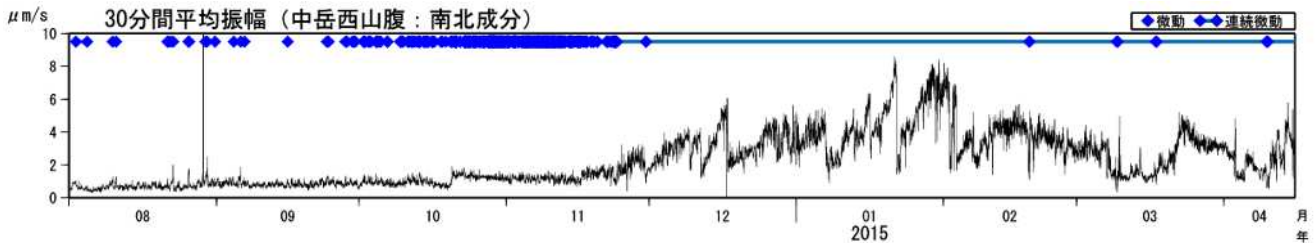
図5 阿蘇山 火山性微動の30分間平均振幅(2014年8月1日～2015年4月16日)
