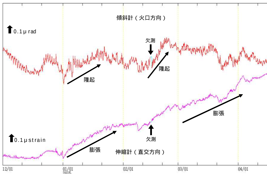
図7 桜島 有村観測坑道の傾斜変動と伸縮変動（2014年12月1日～2015年4月16日）
