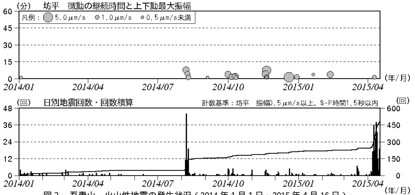
図2 吾妻山 火山性地震の発生状況（2014年1月1日～2015年4月16日）
