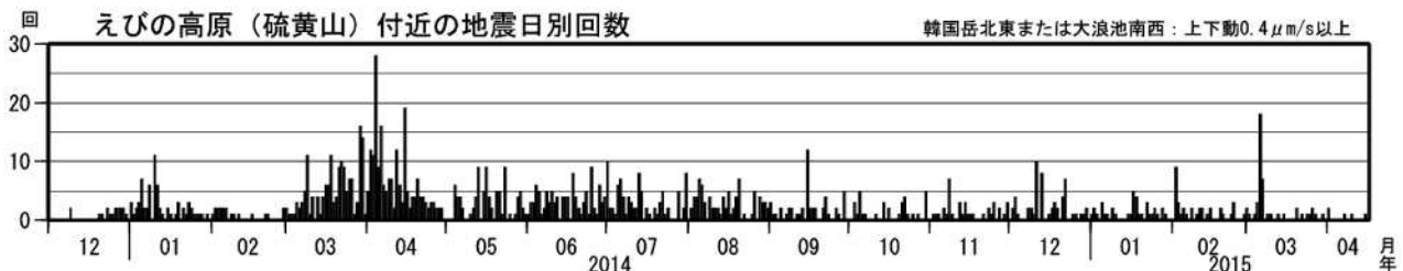
図6 霧島山(えびの高原(硫黄山)周辺) 火山性地震の日別回数 (2013年12月1日～2015年4月16日)
