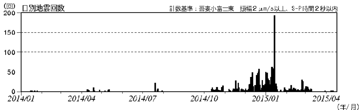
図3 吾妻山 火山性地震の発生状況（2014年1月1日～2015年4月16日）
