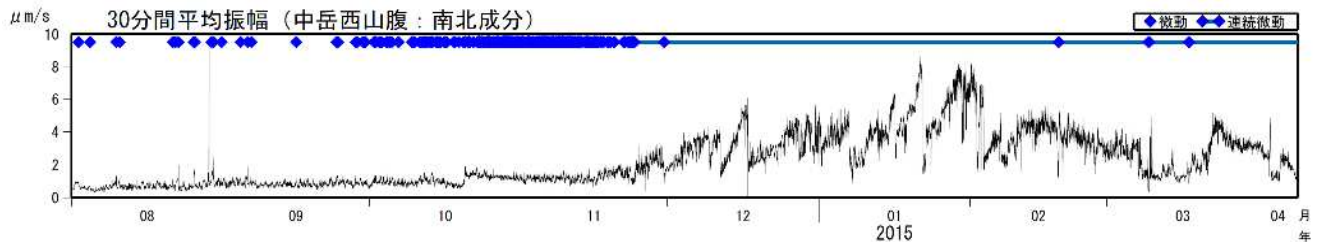
図4 阿蘇山 火山性微動の 30 分間平均振幅 (2014 年 8 月 1 日～2015 年 4 月 9 日)
