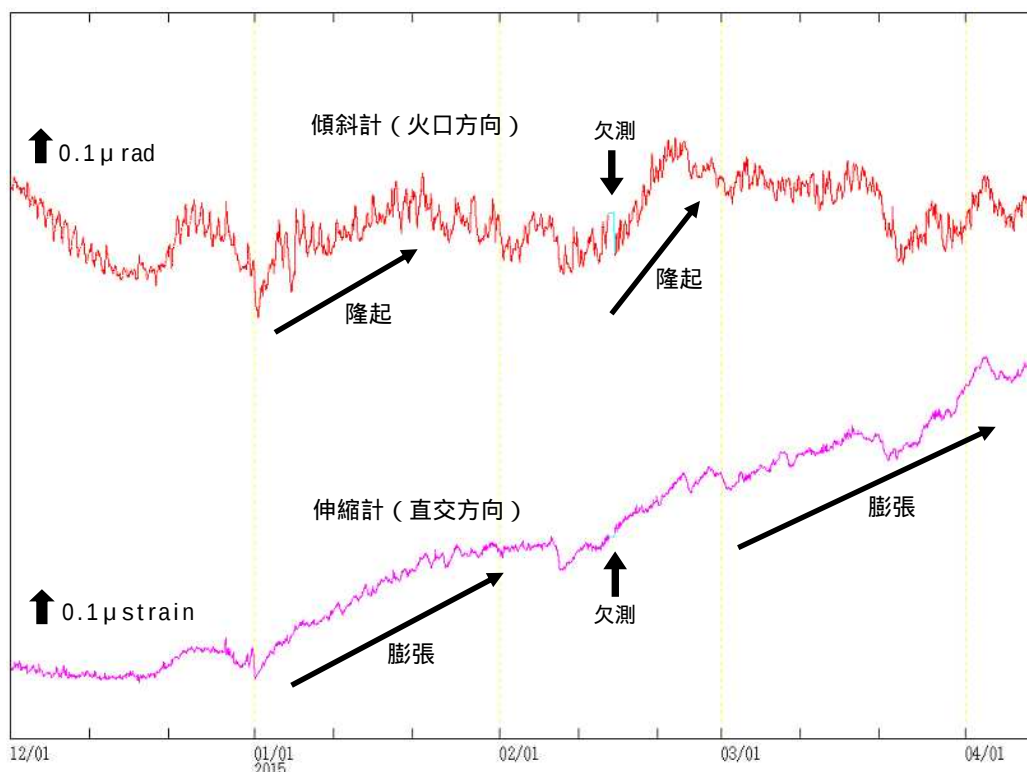
図6 桜島 有村観測坑道の傾斜変動と伸縮変動（2014年12月1日～2015年4月9日）
