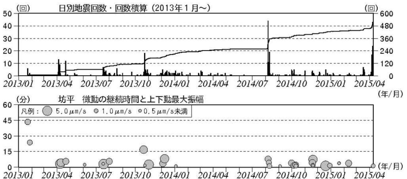
図7 蔵王山 火山性地震の日別回数、火山性微動の発生状況（2013年1月1日～2015年4月9日）
