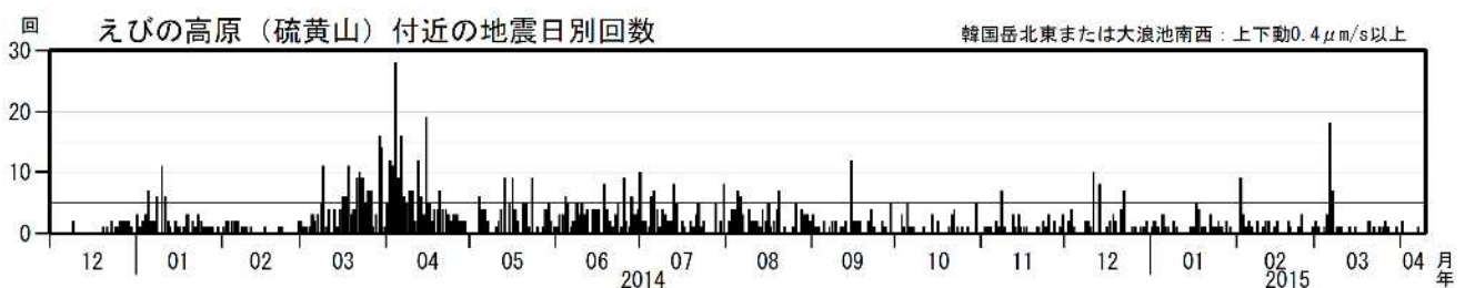
図5 霧島山（えびの高原（硫黄山）周辺） 火山性地震の日別回数 (2013 年 12 月 1 日～2015 年 4 月 9 日)
