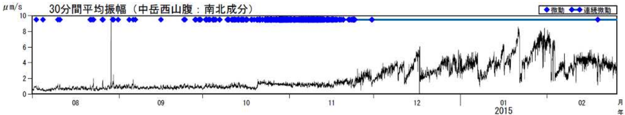
図5 阿蘇山 火山性微動の30分間平均振幅（2014年8月1日～2015年2月26日）
