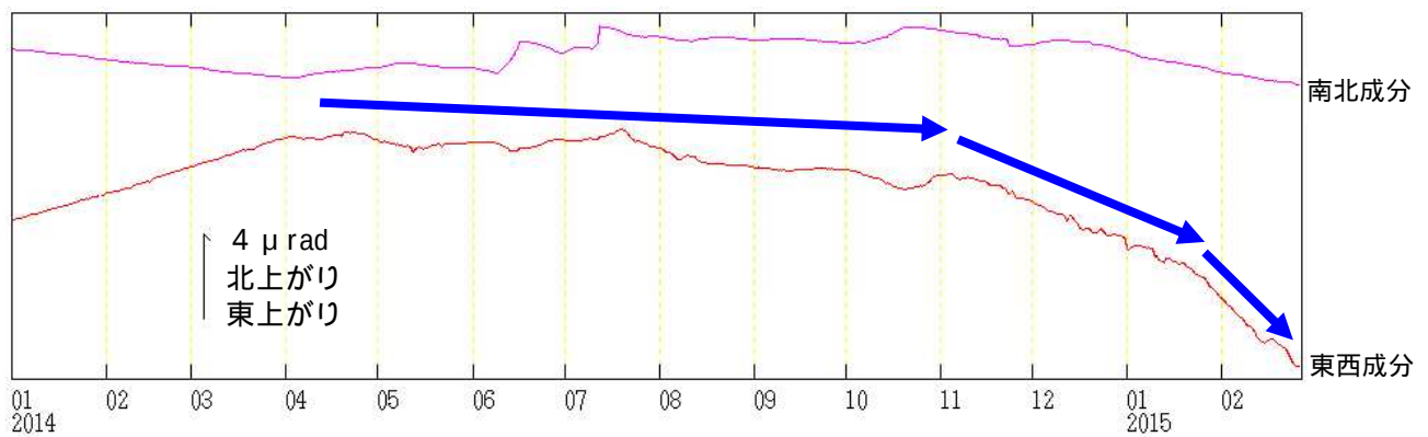
図3 吾妻山 浄土平観測点での傾斜変動（2014年1月1日～2015年2月26日）
