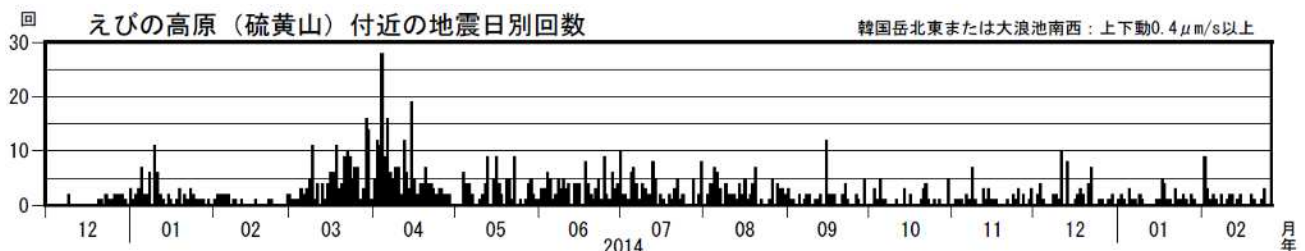
図6 霧島山（えびの高原（硫黄山）周辺） 火山性地震の日別回数 （2013年12月1日～2015年2月26日）
