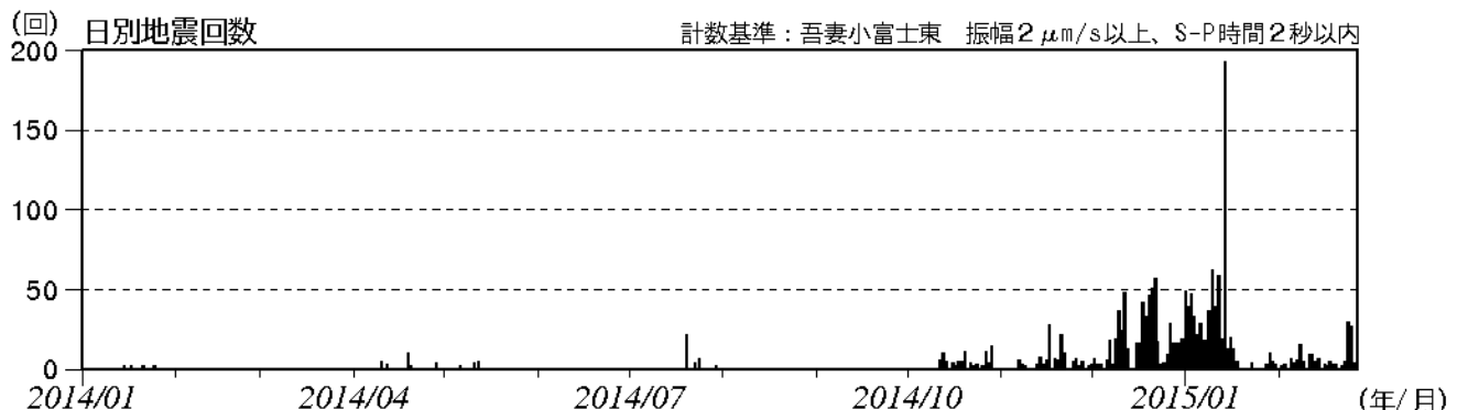
図2 吾妻山 火山性地震の発生状況（2014年1月1日～2015年2月26日）
