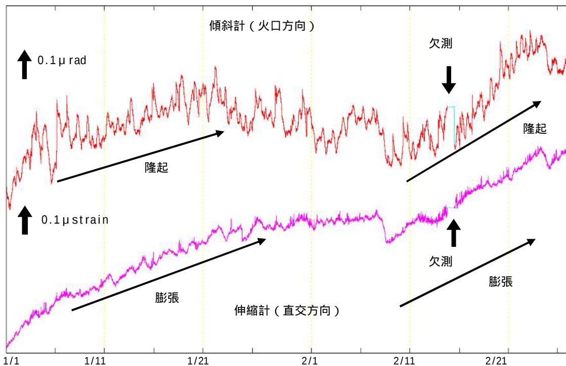
図7 桜島 有村観測坑道の傾斜変動と伸縮変動(2015年1月1日～2015年2月26日)
