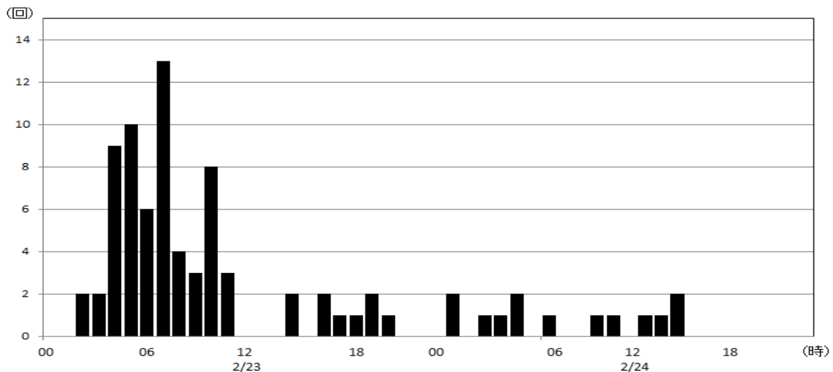
図4 草津白根山 時間別地震回数（2月23日00時～24日24時）
