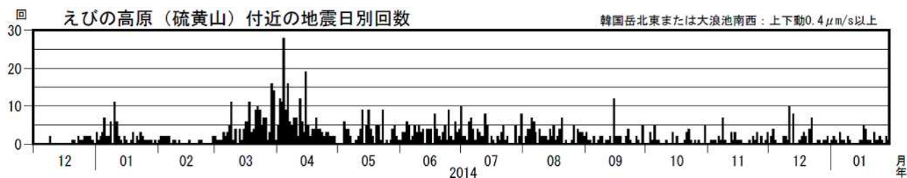
図4 霧島山（えびの高原（硫黄山）周辺） 火山性地震の日別回数 （2013年12月1日～2015年1月29日）
