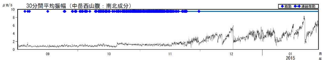
図 3 阿蘇山 火山性微動の 30 分間平均振幅（2014 年 9 月 1 日～2015 年 1 月 29 日）
