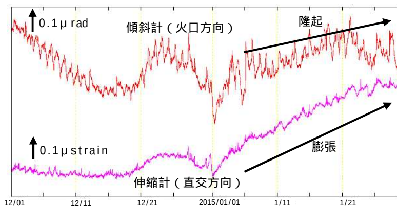
図5 桜島 有村観測坑道の傾斜変動と伸縮変動（2014年12月1日～2015年1月29日）
