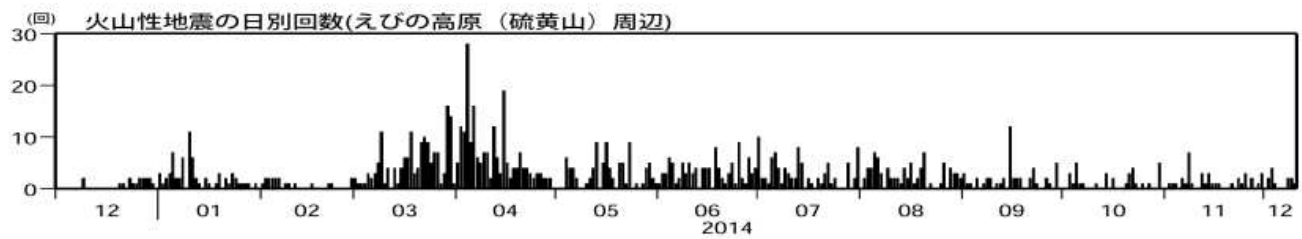
図3 霧島山（えびの高原（硫黄山）周辺） 火山性地震の日別回数 （2013年12月1日～2014年12月11日）
