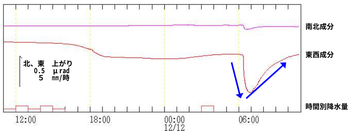
図4 吾妻山 浄土平観測点の傾斜変動（2014年12月11日11時～12月12日11時）
