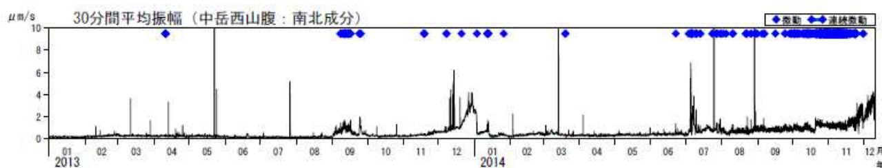
図2 阿蘇山 火山性微動の30分間平均振幅（2013年1月1日～2014年12月11日）
