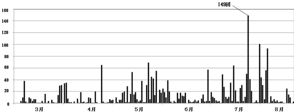
図2 草津白根山 日別地震回数（3月1日～8月21日）
