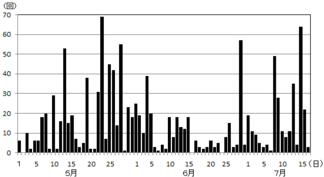
図2 草津白根山 日別地震回数（5月1日～7月17日）
