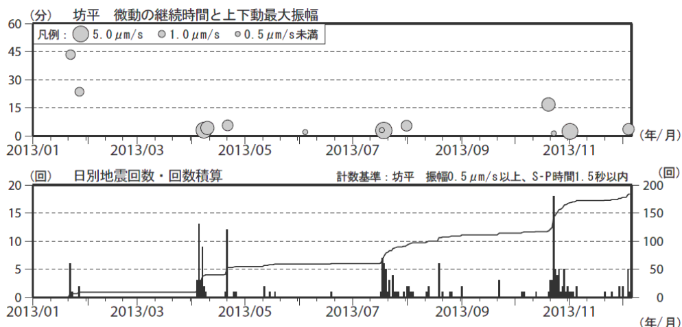
図3 蔵王山 火山性微動と火山性地震の発生状況（2013年1月1日～12月5日）
