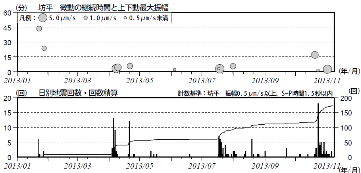
図2 蔵王山 火山性微動と火山性地震の発生状況（2013年1月1日～11月7日）
