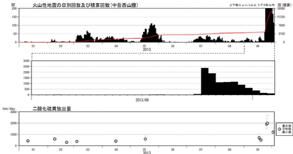
図2 阿蘇山 火山性地震の発生状況および二酸化硫黄の放出量（2013年1月1日～2013年10月3日）
