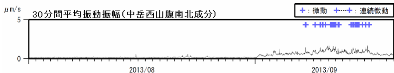
図2 阿蘇山 火山性微動の発生状況(2013年8月1日~2013年9月19日)
