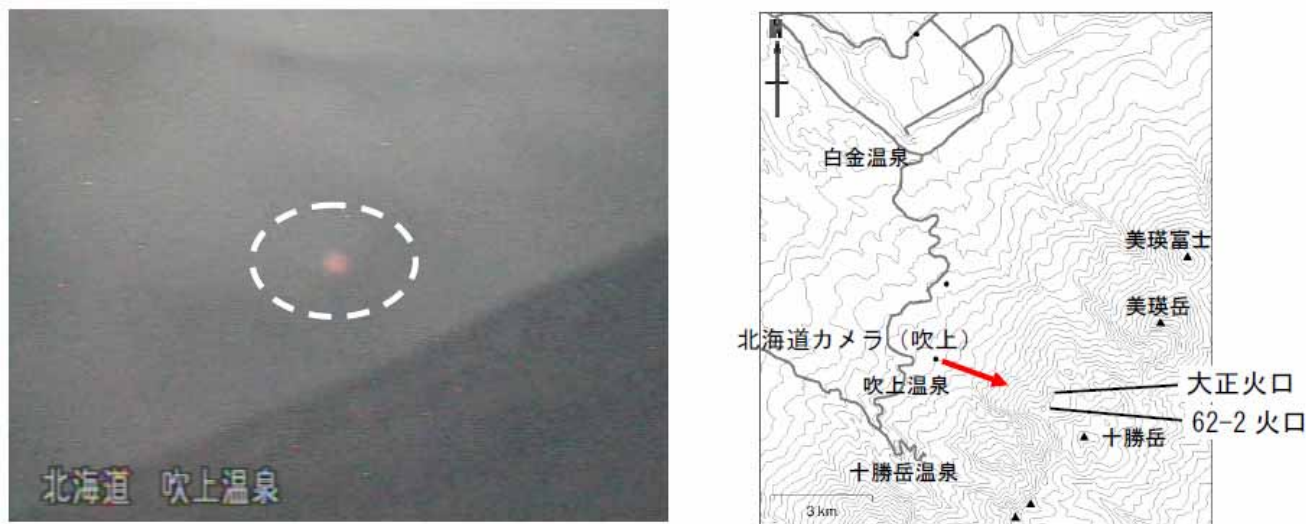
図 2 十勝岳 大正火口付近が明るく見える現象と遠望カメラ位置及び撮影方向（赤矢印）
