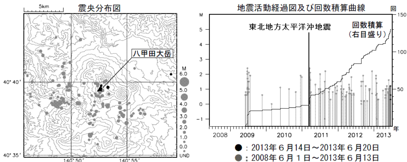
図2 八甲田山 広域地震観測網による山頂付近及び周辺の地震活動（2008年6月1日～2013年6月20日）
