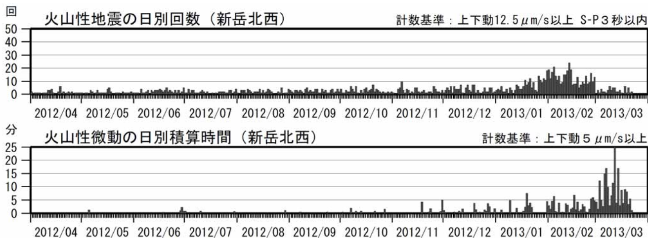
図2 口永良部島 火山性地震の発生回数（2012年4月1日～2013年3月21日）
