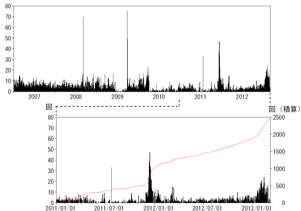
図3 口永良部島 火山性地震の発生回数(2007年1月1日～2013年3月7日)
