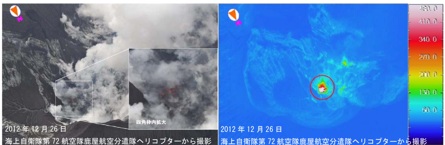
図2 諏訪之瀬島 御岳火口内の状況（左図：可視画像 右図：赤外画像）
