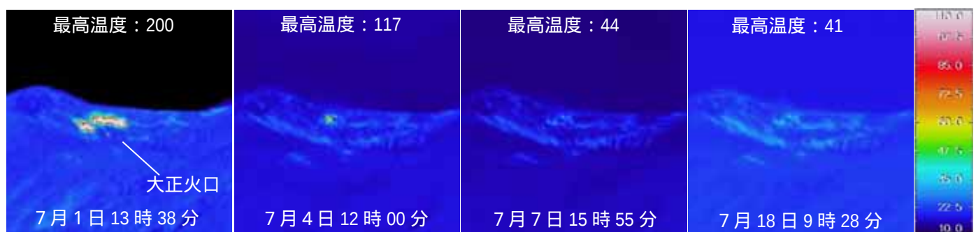
図2 十勝岳 赤外熱映像装置 5) による大正火口の地表面温度分布 (大正火口の北西約3.5kmの地点から撮影した画像を拡大)
