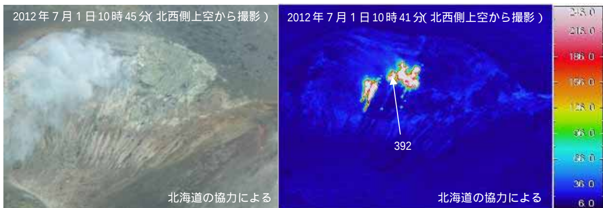
図4 十勝岳 赤外熱映像装置 4) による大正火口及び周辺の地表面温度分布図（北西側上空から撮影）
