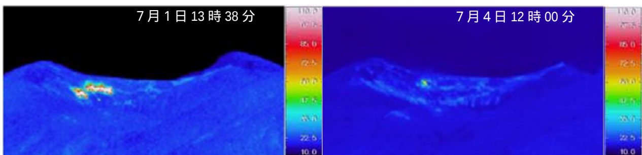
図5 十勝岳 赤外熱映像装置 4) による大正火口及び周辺の地表面温度分布図（火口から3.5kmの富良野川西岸から撮影した画像を拡大）
