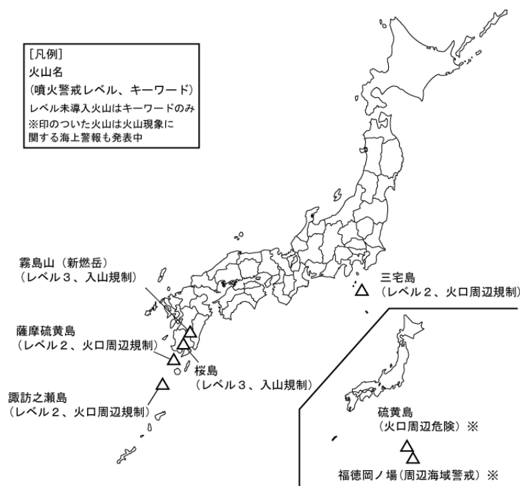
図 1 噴火警報及び火山現象に関する海上警報発表中の火山（5月17日現在）
