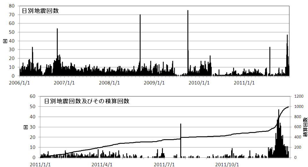
図 2 口永良部島 火山性地震の発生回数（2006 年 1 月 1 日～2011 年 12 月 29 日）
