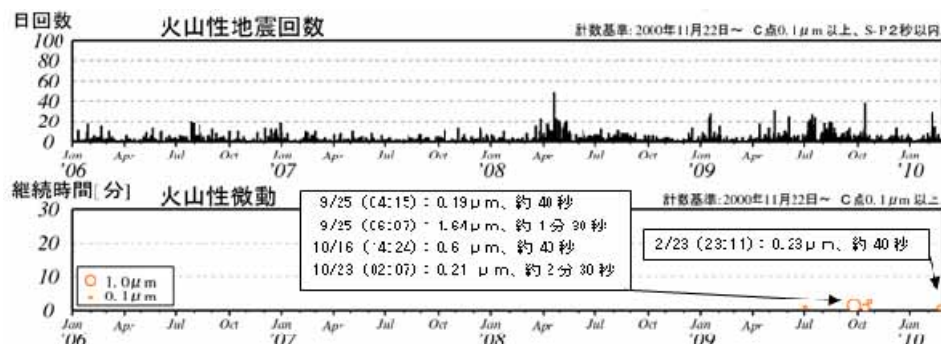
図 2 樽前山 火山性地震と火山性微動の経過グラフ（2006 年 1 月 1 日～2010 年 2 月 25 日）
