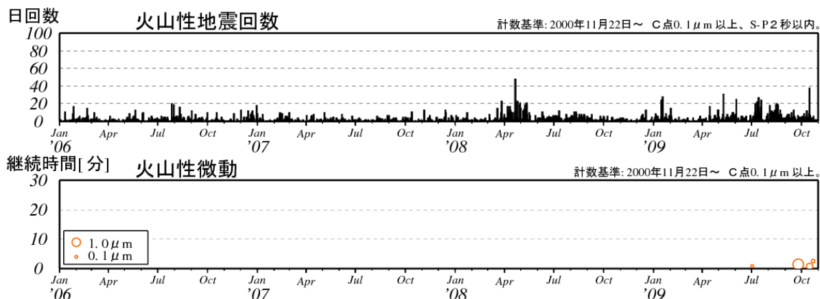
図2 樽前山 火山性地震と火山性微動の経過（2006年1月1日～2009年10月29日）
