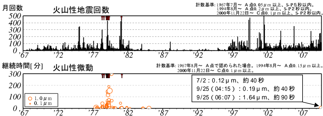
図 2 樽前山 火山性地震と火山性微動の経過グラフ（1967 年 7 月～2009 年 9 月 25 日） ：噴火を示す
