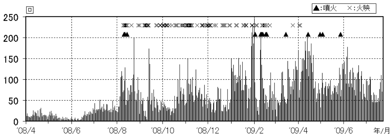
図2 浅間山 火山性地震の日別回数（2008 年 4 月 1 日～2009 年 7 月 23 日）
