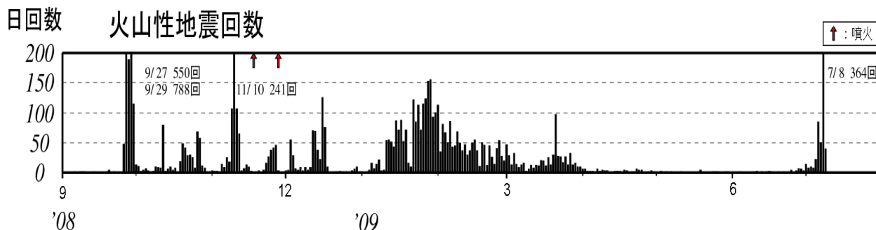
図3 雌阿寒岳 火山性地震の日別回数（2008年9月1日～2009年7月9日）
