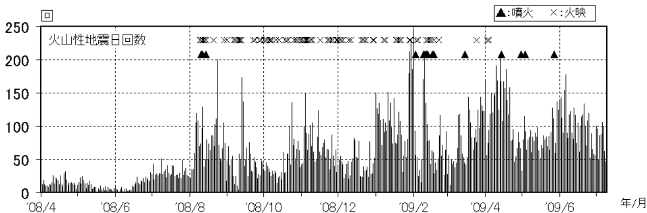
図2 浅間山 火山性地震の日別回数（2008年4月1日～2009年7月9日）
