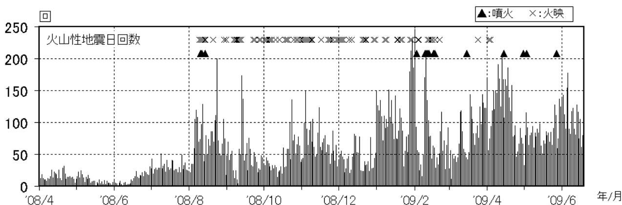
図2 浅間山 火山性地震の日別回数（2008 年4月1日～2009 年6月18日）
