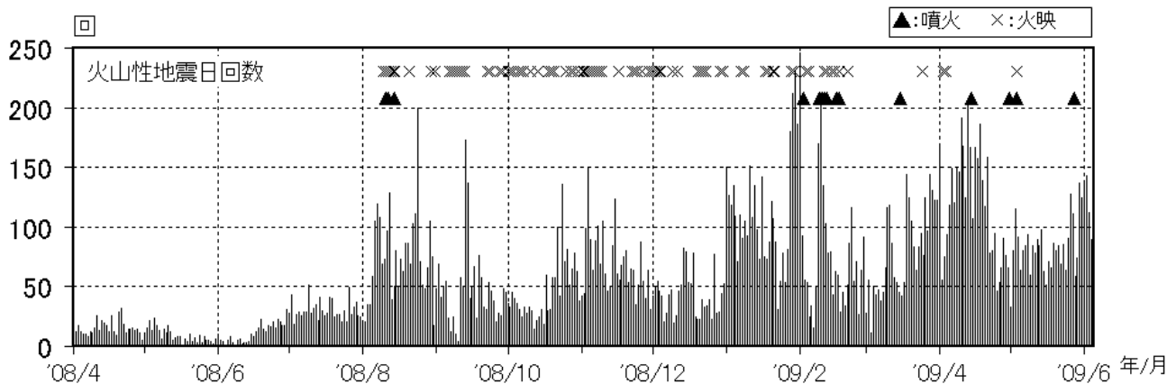
図2 浅間山 火山性地震の日別回数(2008年4月1日～2009年6月4日)
