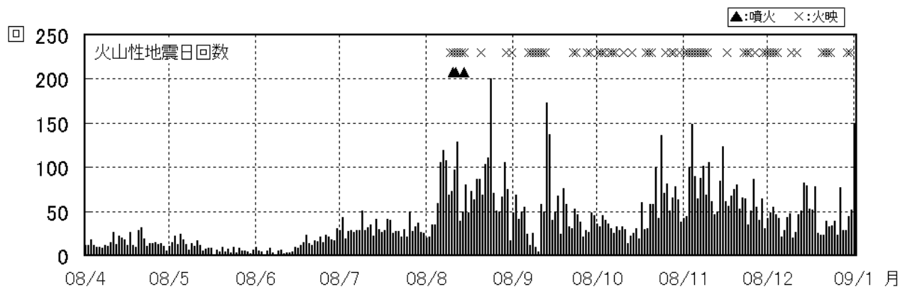
図2 浅間山 火山性地震の日別回数（2008年4月1日～2009年1月1日）
