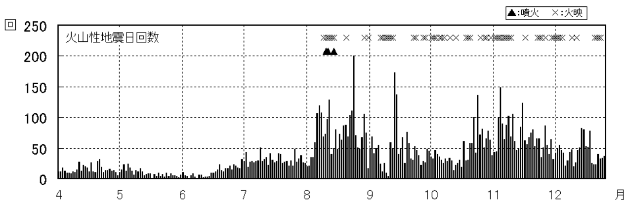
図2 浅間山 火山性地震の日別回数 (2008年4月1日～12月25日)
