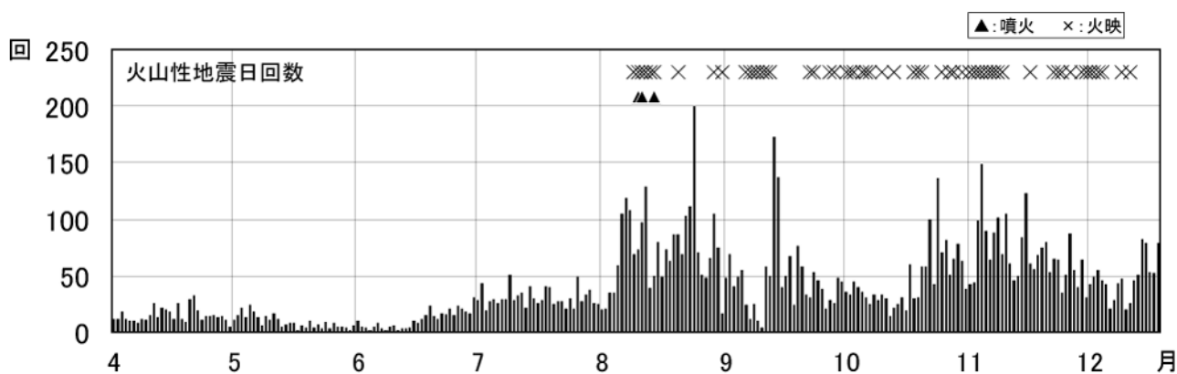
図2 浅間山 火山性地震の日別回数(2008年4月1日～12月18日)
