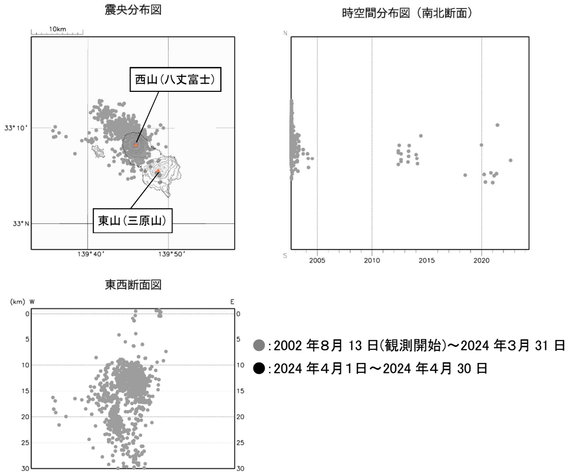
図3 八丈島 震源分布図（2002年8月13日～2024年4月30日）
