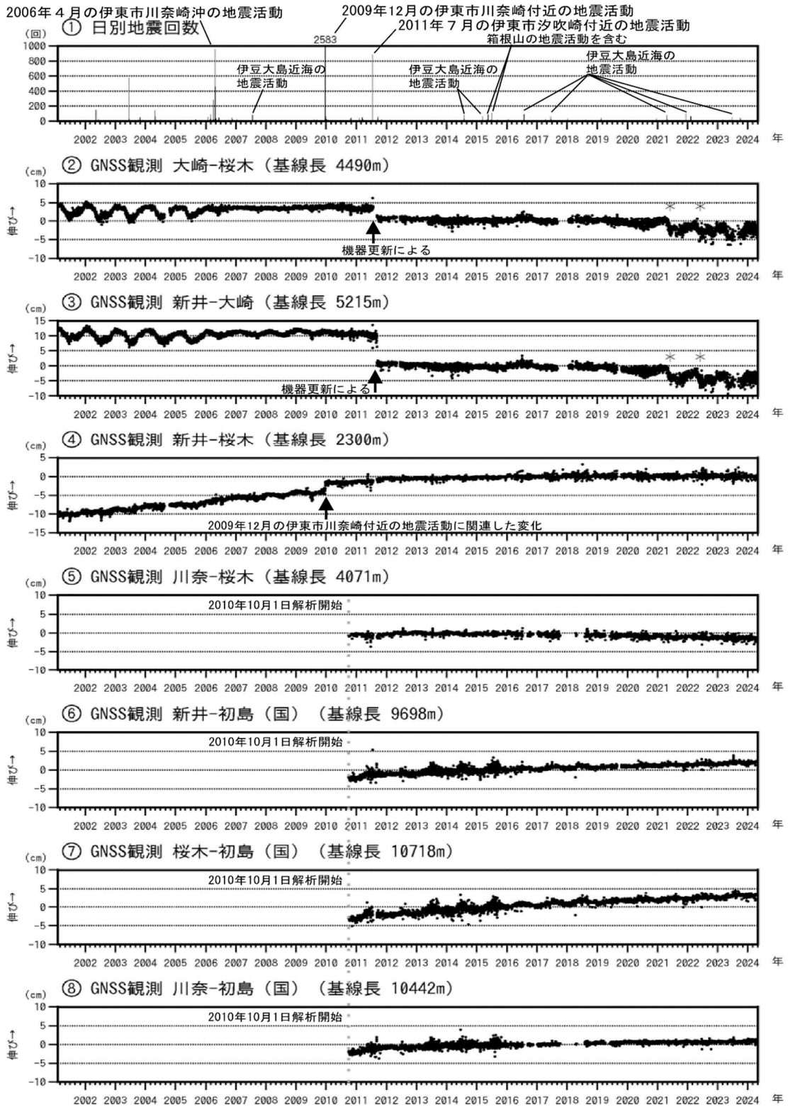
図3 伊豆東部火山群 火山活動経過図 (2001年2月1日~2024年4月30日)
