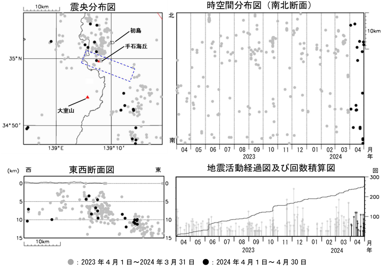
図2 伊豆東部火山群 広域地震観測網による震源分布図（2023年3月1日～2024年4月30日） □の領域は群発地震活動の発生する可能性がある範囲（火口が出現する可能性のある範囲）を示しています。 https://www.data.jma.go.jp/vois/data/tokyo/STOCK/level/PDF/level_316.pdf 広域地震観測網により震源決定したもので、深さは全て海面以下として決定しています。 M（マグニチュード）は地震の規模を表し、M0.0以上を表示しています。 図中の震源要素は一部暫定値が含まれており、後日変更することがあります。 この図では、関係機関の地震波形を一元的に処理し、地震観測点の標高を考慮する等した手法で得られた震源を用いています。
