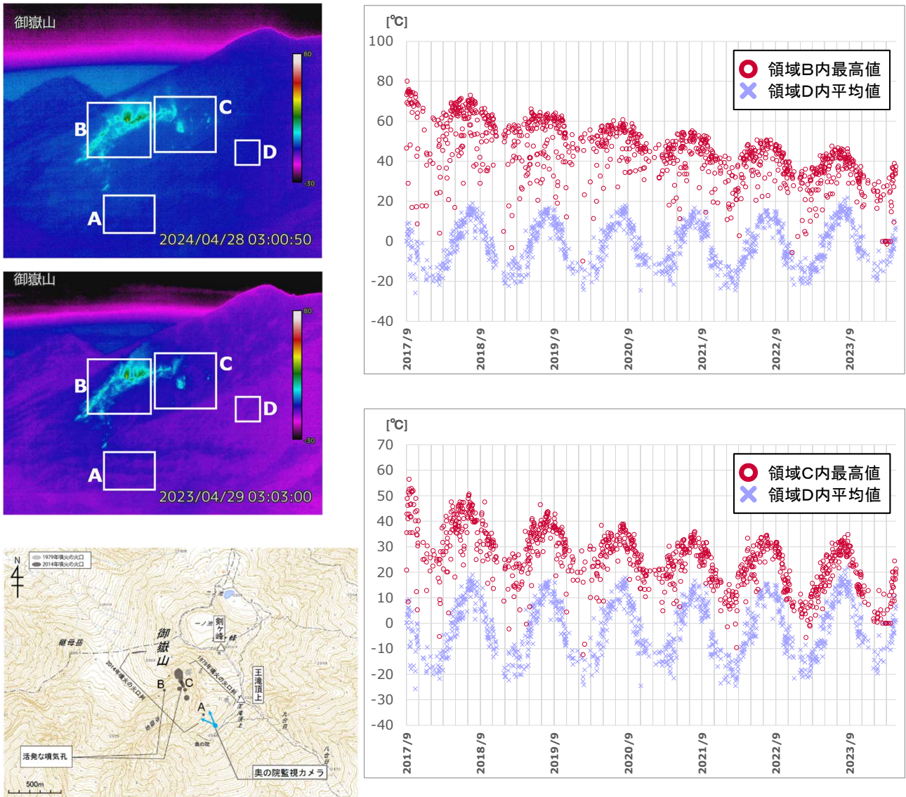
図3 御嶽山 奥の院赤外熱映像カメラによる剣ヶ峰南西側における最高温度の推移 (2017年9月13日～2024年4月30日)
