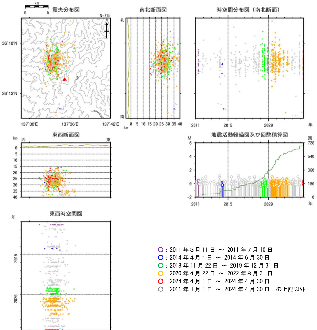
図10 焼岳 広域地震観測網による深部低周波地震の震源分布図（2011年1月1日～2024年4月30日） 広域地震観測網により震源決定したもので、深さは全て海面以下として決定しています。そのため、山頂付近の浅い地震の震源も海面下に決定されています。 M（マグニチュード）は地震の規模を表します。 図中の震源要素は一部暫定値が含まれており、後日変更することがあります。 ・ 焼岳の北西側の深い所を震源とする低周波地震は引き続き観測されており、中旬にやや増加しました。この活動に伴う焼岳周辺の地震活動の活発化はみられません。 ・ 過去には、図9に示したような焼岳周辺の地震活動の活発化がみられた期間付近で、深部低周波地震が増加したことがあります。
