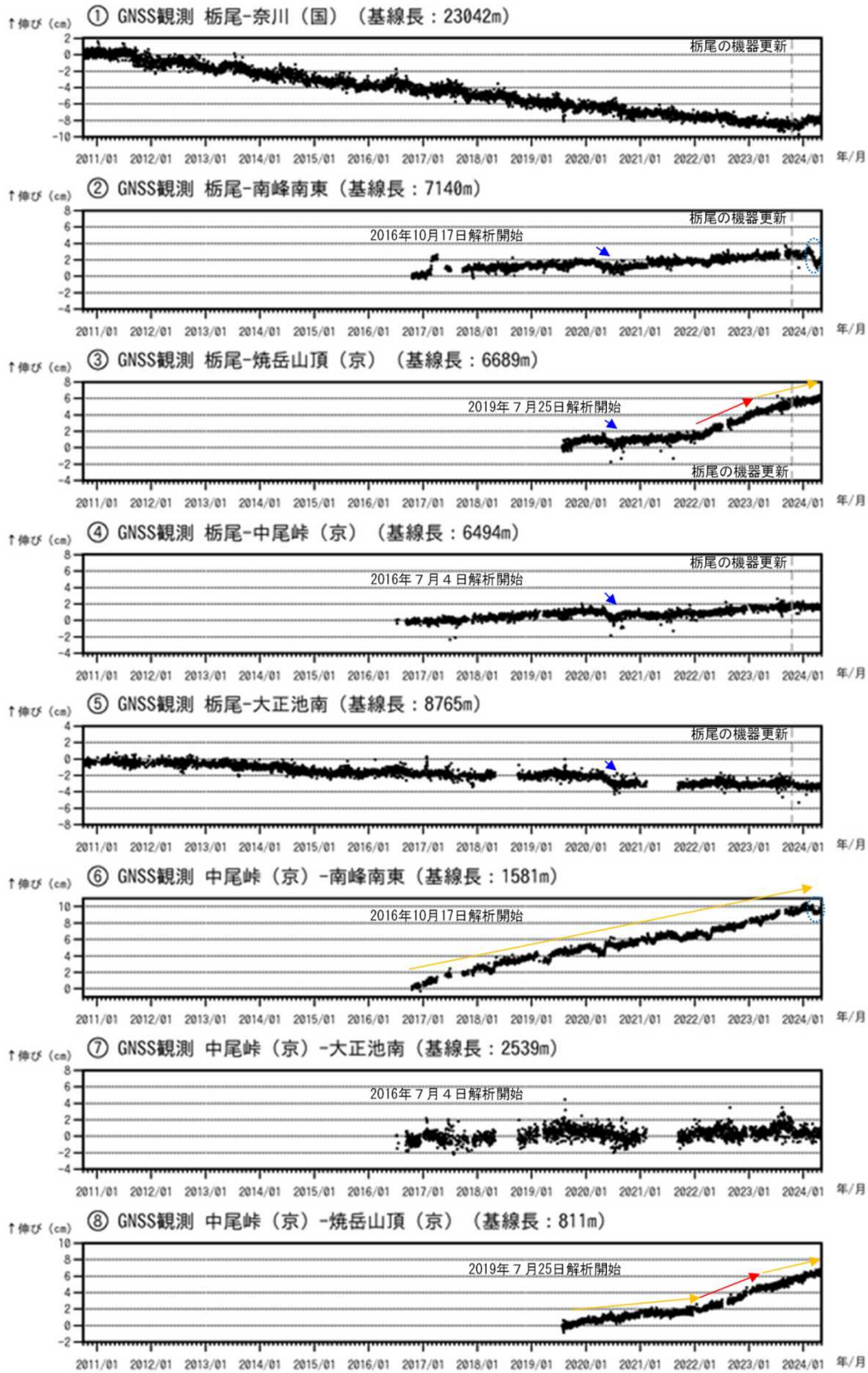
図6 焼岳 GNSS 連続観測による基線長変化（2010年10月1日～2024年4月30日）
