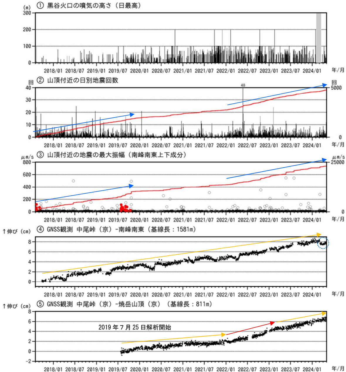
図1 焼岳 火山活動経過図（2017年8月1日～2024年4月30日）
