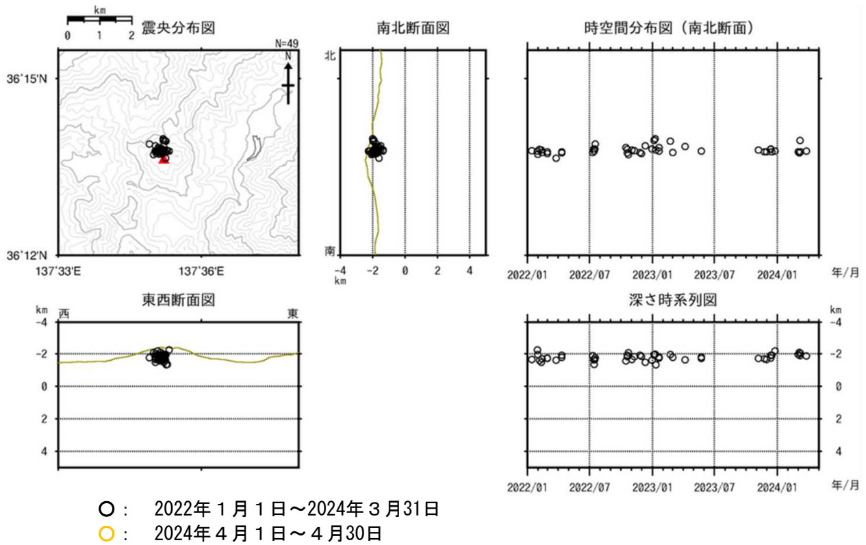
図2 焼岳 山頂付近の地震の震源分布図（2022年1月1日～2024年4月30日）
