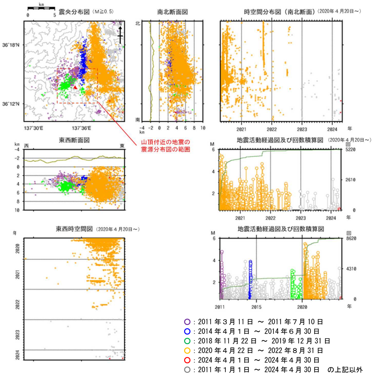
図9 焼岳 広域地震観測網による山体及び周辺の地震活動(2011年1月1日～2024年4月30日)
