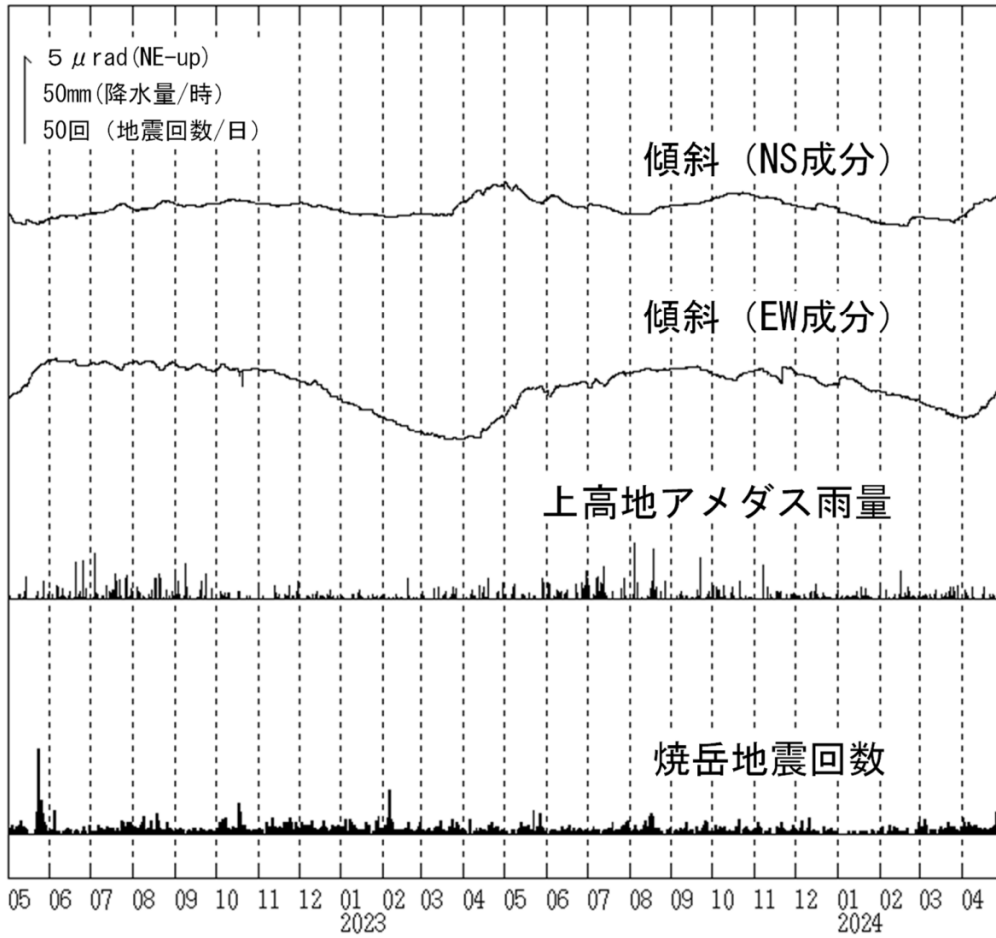
図8 焼岳 南峰南東観測点における傾斜データ（2022年4月1日～2024年4月30日） ・傾斜計による観測では、火山活動によるとみられる変動は認められません。
